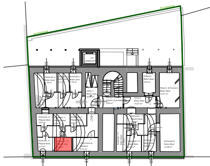
Kellergeschoß 1:500
