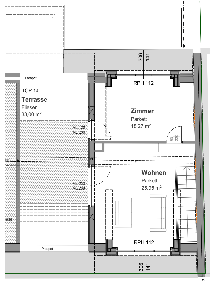
Empore 1:100
